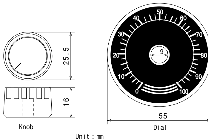
Unit : mm
